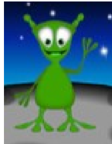
alien
