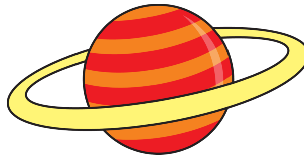
planet
